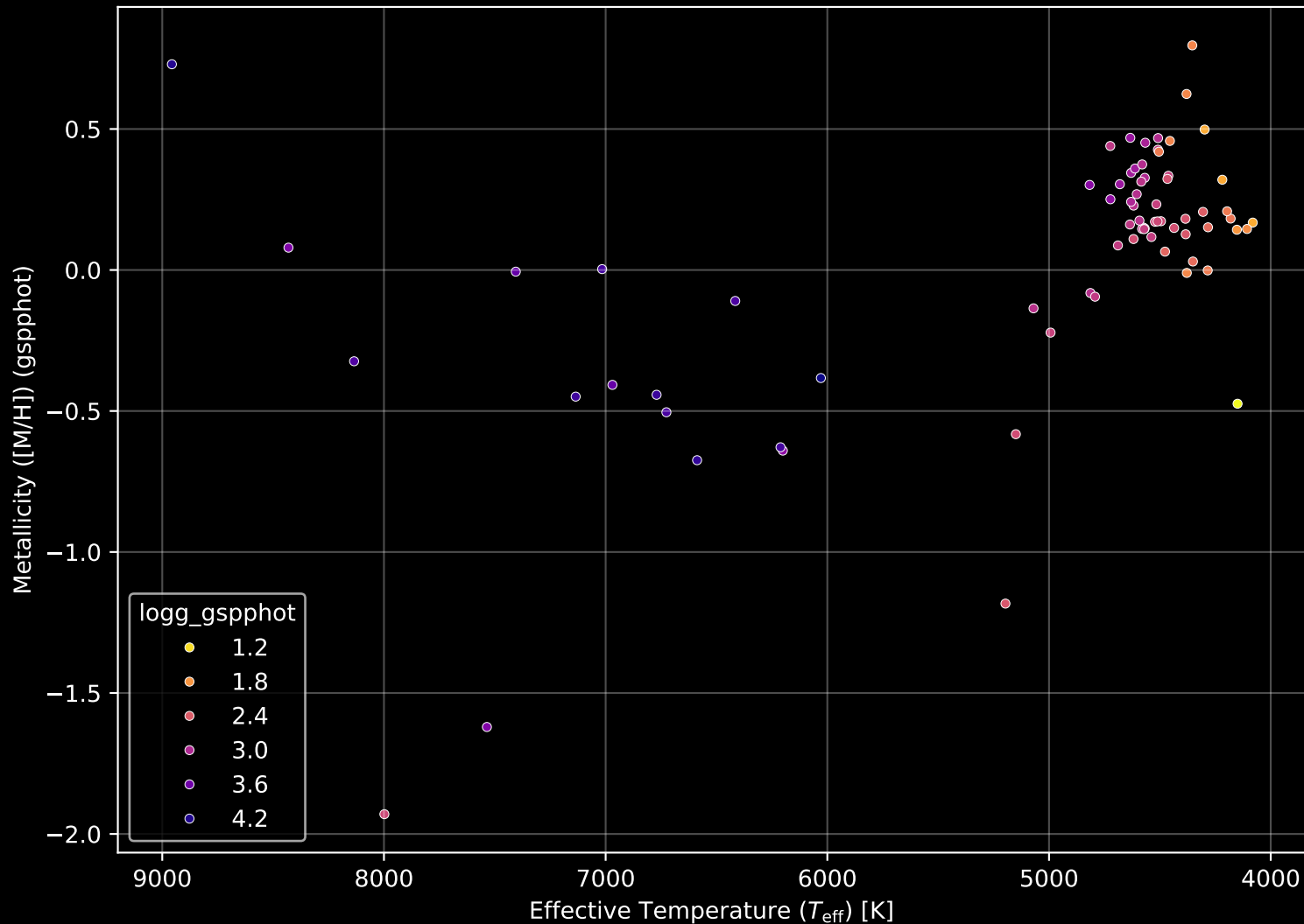
APOGEE DR17 Field: [LMC30] Stellar Population Parameters (n= 74)
